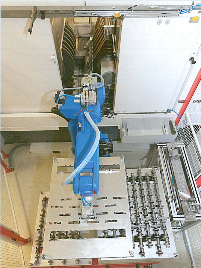
Nach der überzeugenden Automation der 35 Jahre alten Lidköping Anfang 2010 orderte Lerchenmüller auch für die Ende 2010 installierte Mikrosa Kronos L660 bei FMB eine schlüsselfertige Unirobot Automationszelle. Markant sind bei beiden Lösungen die ausgeklügelten Werkstückaufnahmeplatten für die lagefeste Aufnahme von jeweils 10 respektive 8 Exzenterwellen.
